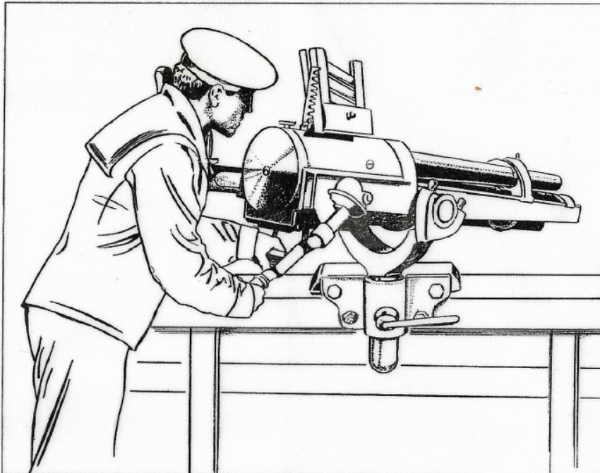
Skjydning med 37 mm revolverkanon placeret i lønningsbeslag. (Tegnet af Kirsten Yde-Andersen, TM).
